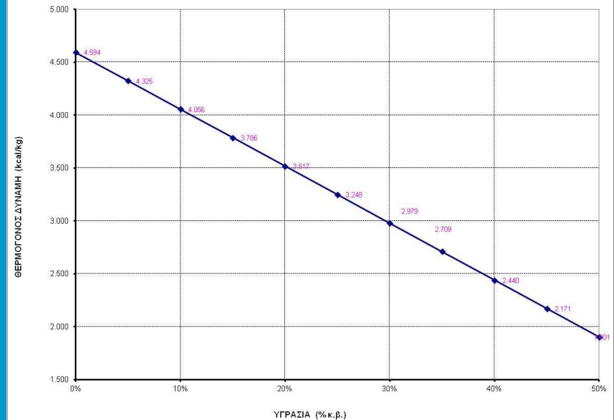
ΔΙΑΓΡΑΜΜΑ ΘΕΡΜΟΓΟΝΟΥ ΔΥΝΑΜΗΣ ΒΙΟΜΑΖΑΣ ΜΕ ΠΕΡΙΕΧΟΜΕΝΗ ΥΓΡΑΣΙΑ
