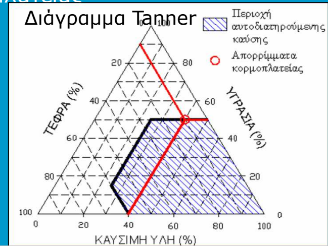
ΔΙΑΓΡΑΜΜΑ ΘΕΡΜΟΓΟΝΟΥ ΔΥΝΑΜΗΣ ΒΙΟΜΑΖΑΣ ΜΕ ΠΕΡΙΕΧΟΜΕΝΗ ΥΓΡΑΣΙΑ
